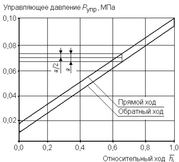
Рисунок 1 – Диаграмма определения нечувствительности регулирующей арматуры «НО» с ПИМ, для диапазона управляющего давления P_{упр} от 0,02 до 0,1 МПа
