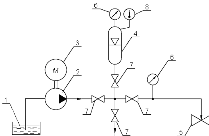
Рисунок В.4 – Принципиальная схема стенда для количественного определения утечек в затворе арматуры с применением манометрического метода контроля (способ реализации метода – компрессионный)
